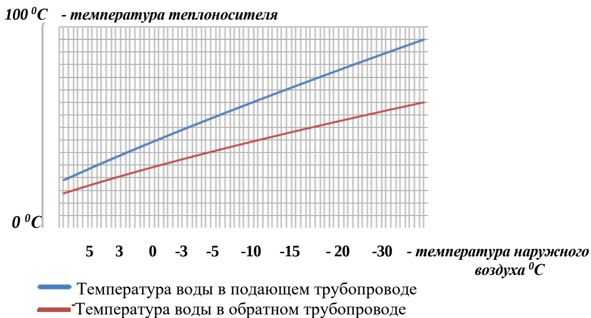
Рис. № 5 - Температурный график качественного регулирования 95/70 °С
