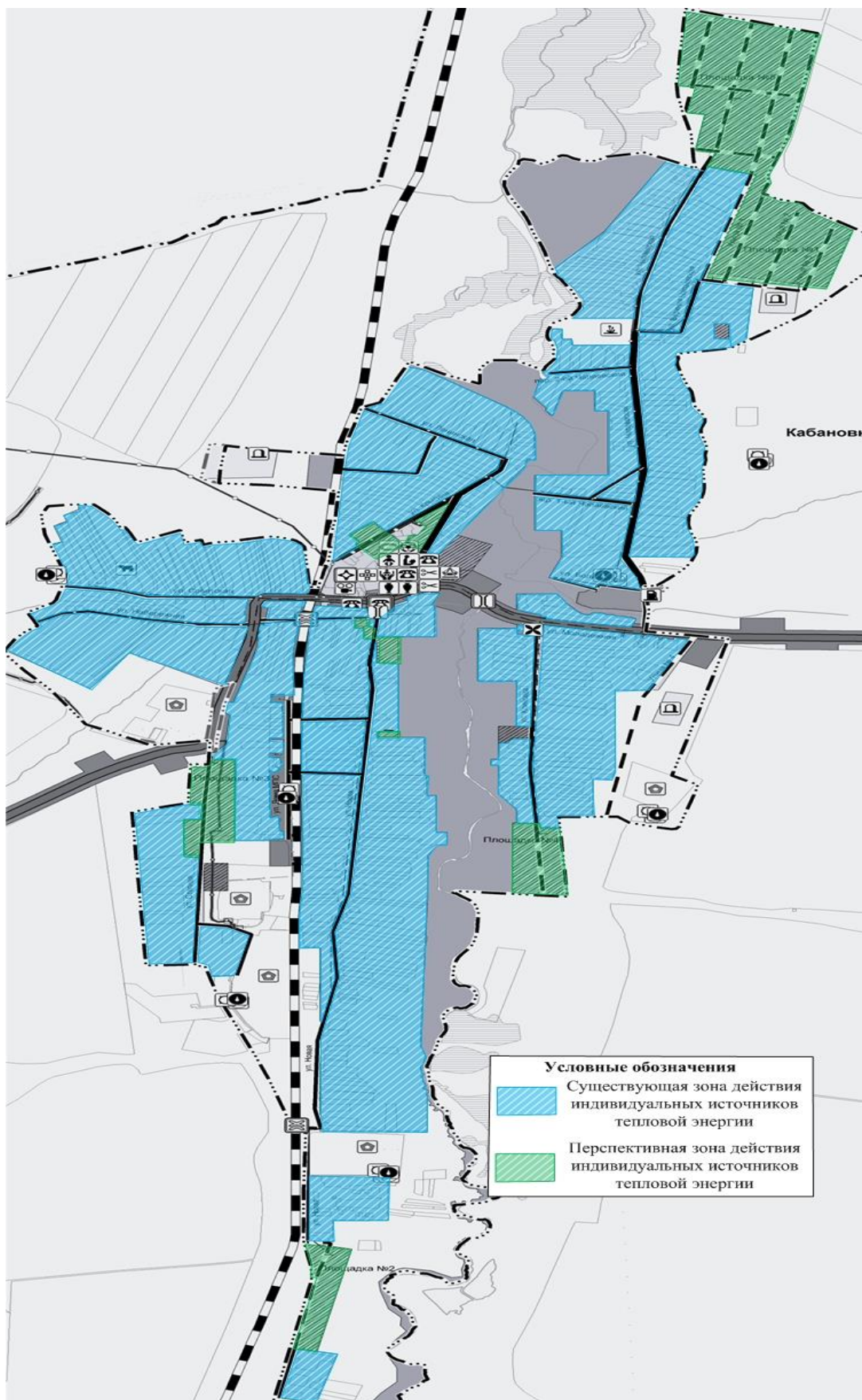
Рис. № 26 - Существующие и перспективные зоны действия индивидуальных источников тепловой энергии на территории села Кabanовка
