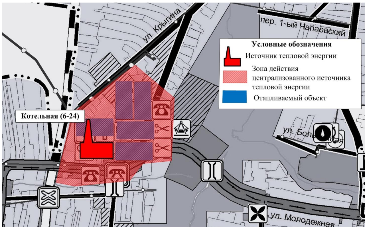
Рис. № 8 - Зона действия централизованного источника тепловой энергии на территории с. Кабановка
