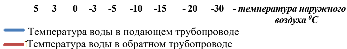
Рис. № 5 - Температурный график качественного регулирования 95/70 °С
