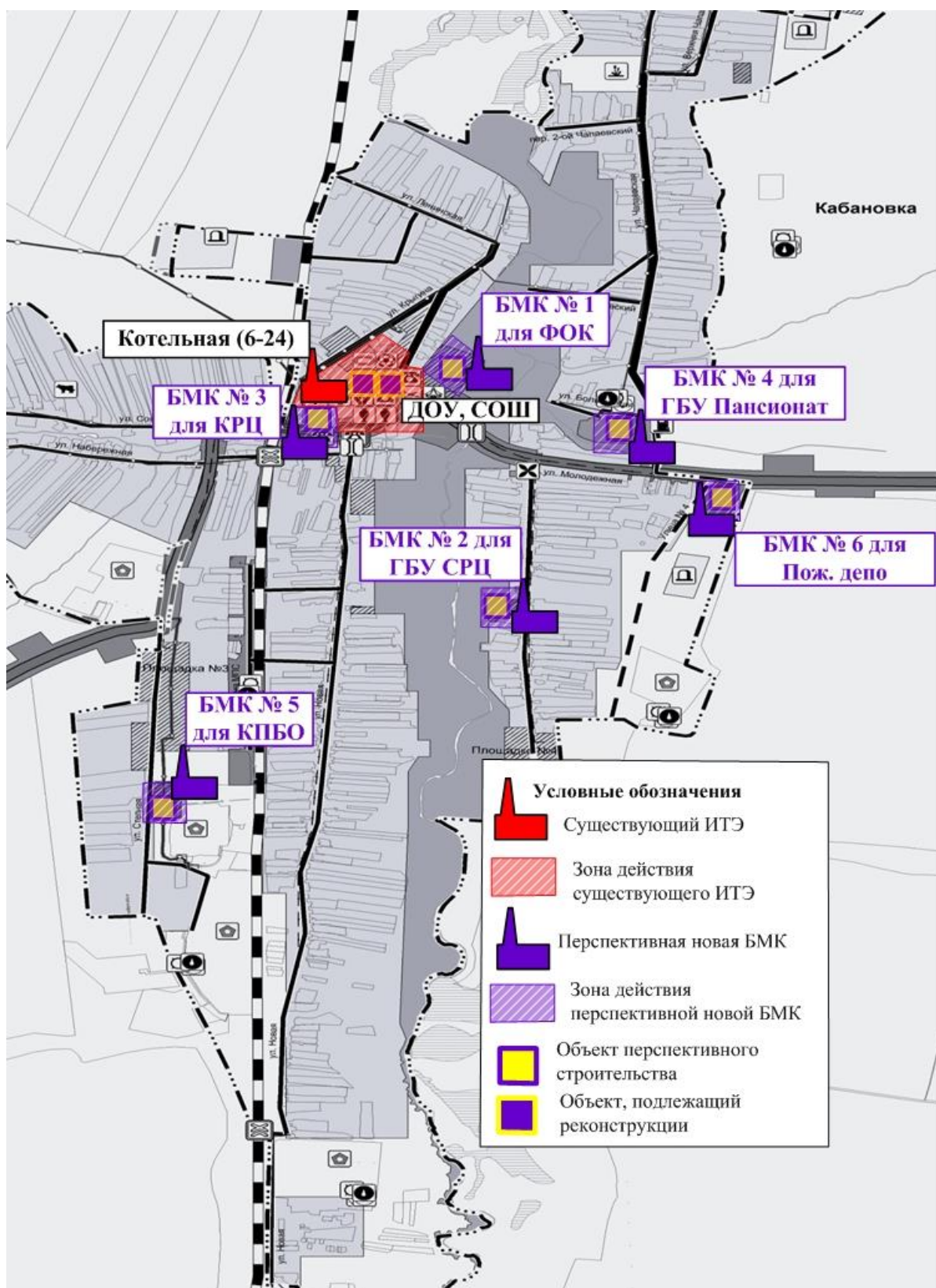
Рис. № 23 - Перспективные зоны теплоснабжения существующей котельной и блочно-модульных источников тепловой энергии, планируемых к размещению на территории села Кабановка
